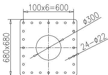
起重机底板安装尺寸
