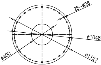
起重机底板安装尺寸
