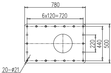
起重机底板安装尺寸
