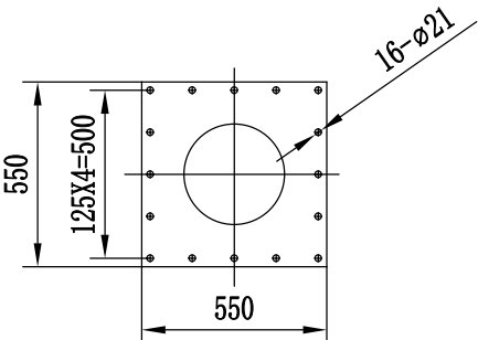
起重机底板安装尺寸
