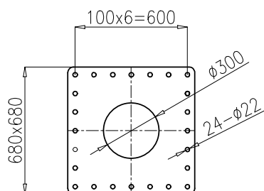
起重机底板安装尺寸
