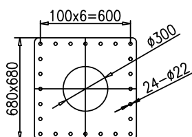
起重机底板安装尺寸
