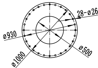
起重机底板安装尺寸
