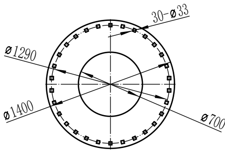
起重机底板安装尺寸
