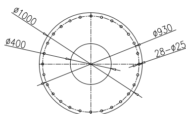
起重机底板安装尺寸
