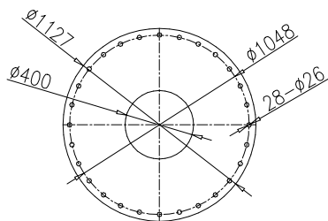
起重机底板安装尺寸
