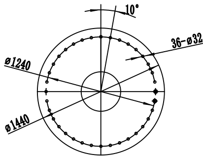
起重机底板安装尺寸
