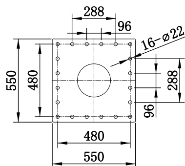
起重机底板安装尺寸
