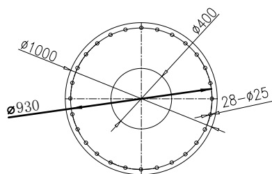
起重机底板安装尺寸
